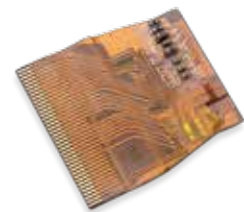
Small F-PCB Module
